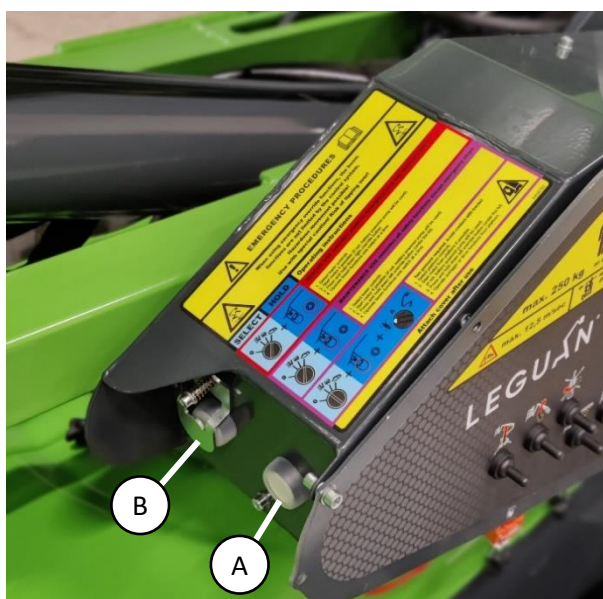
Figur 13. Tilsidesættelsesknapper
