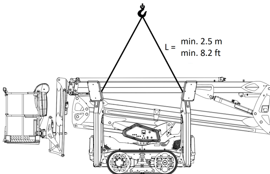
Figur 14. Løft af adgangsplatformen
