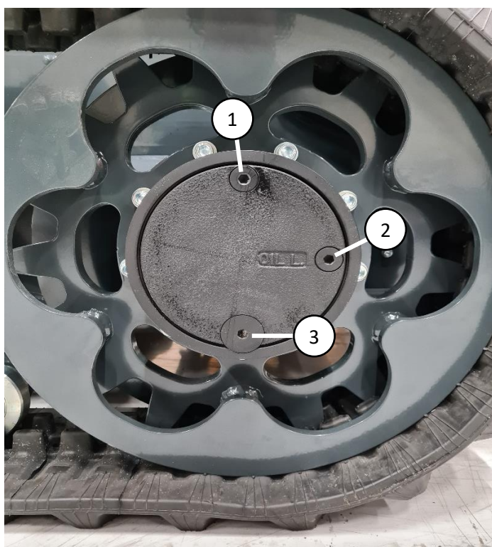
Figur 29. Skift af gearolie i drivmotor
