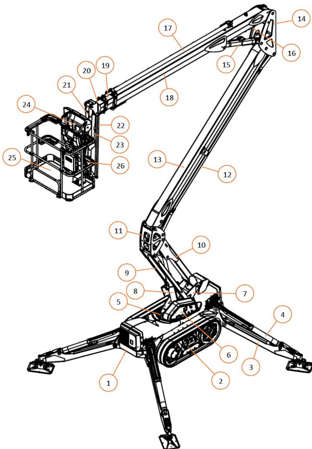
Figur 1. Hoveddele
