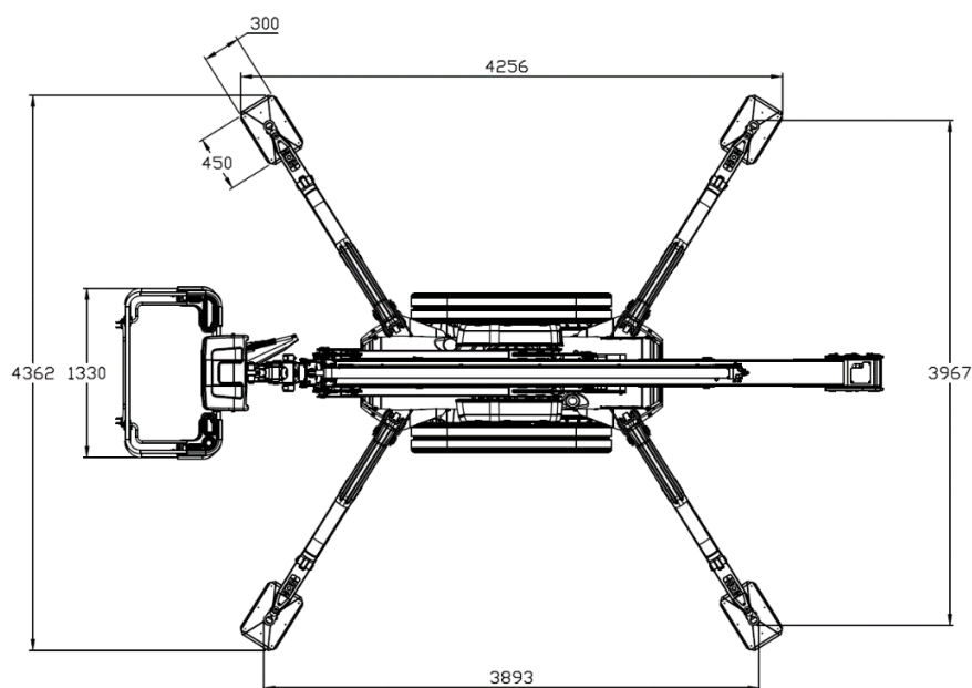
Figur 2. Krævet plads til støtteben i yderste position
