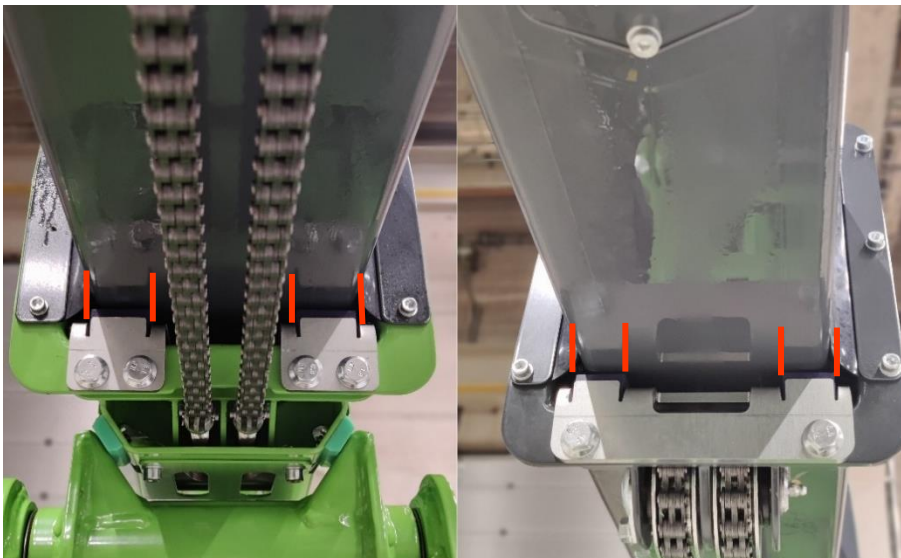
Abbildung 24. Breite der gefetteten Fläche am mittleren Ausleger und an der Verlängerung mit roten Linien hervorgehoben
