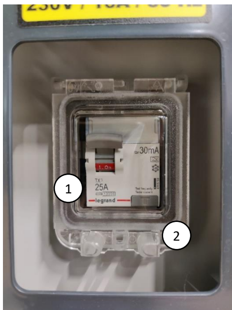
Abbildung 12. Fehlerstrom-Schutzeinrichtung
