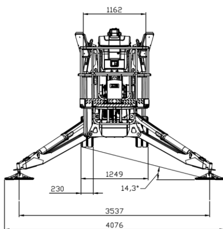
Abbildung 4. Hauptabmessungen von hinten
