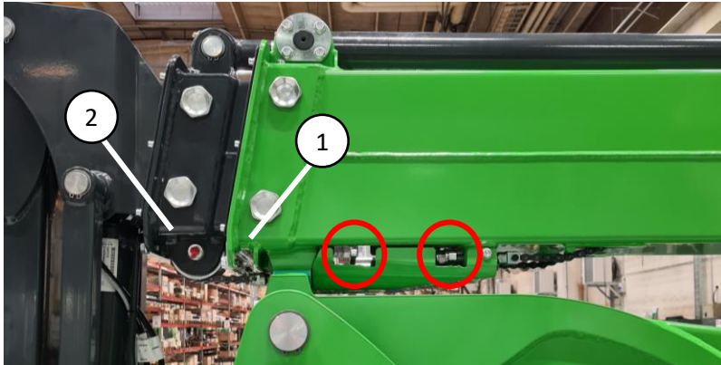
Abbildung 17. Anzeiger der Teleskopkettenspannung
