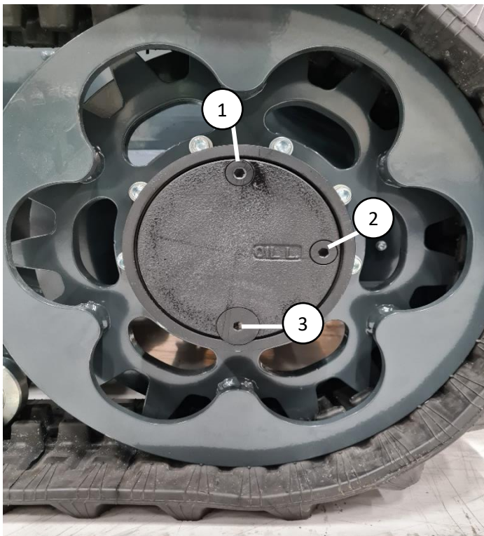
Abbildung 29. Getriebeölwechsel beim Antriebsmotor
