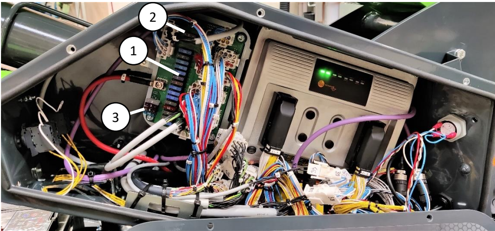
Abbildung 44. Sicherungen der Zugangsplattform
