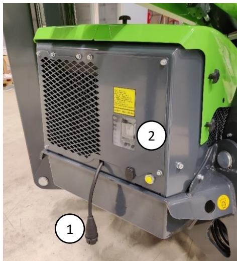
Abbildung 11. 230 V-Anschlüsse
