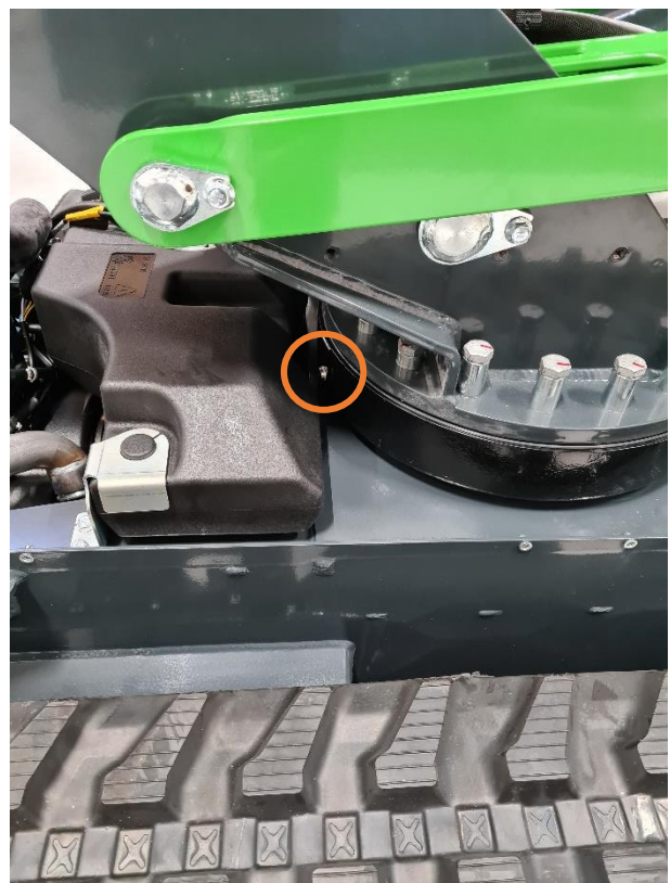
Abbildung 21. Drehkranzschmierung Druckentlastungsschraube
