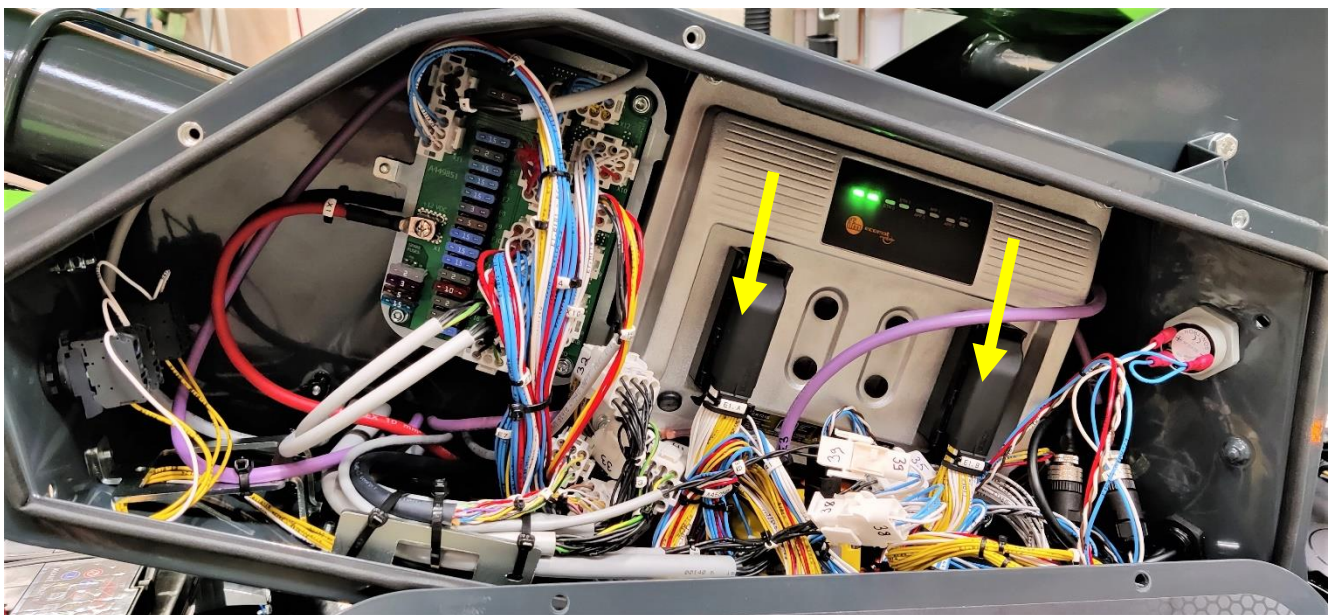
Abbildung 46. Anschlüsse der Logiksteuerung im unteren Steuerkasten
