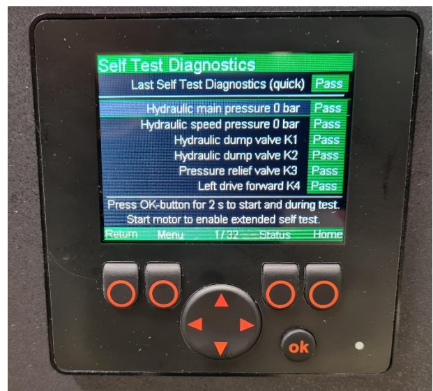
Abbildung 41. Auswahl „Selbsttest Diagnose“
