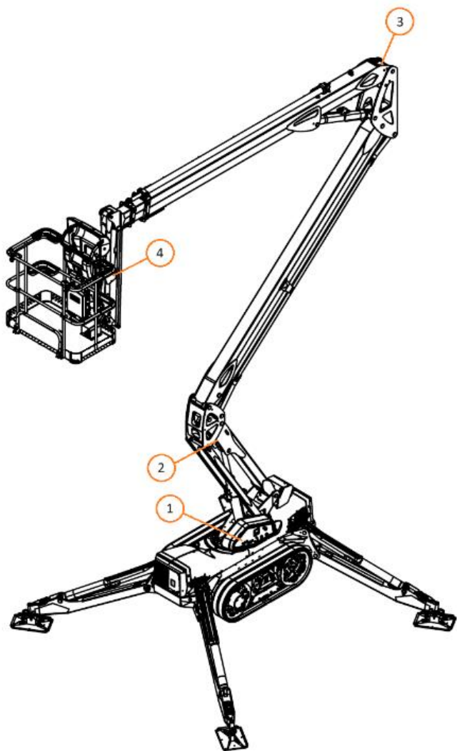
Kuva 38. Nostimen asentoanturit
