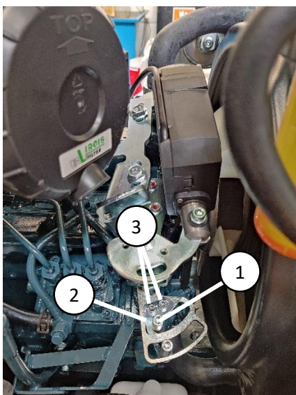
Kuva 28. Kaasunsäätömoottorin minimiasento
