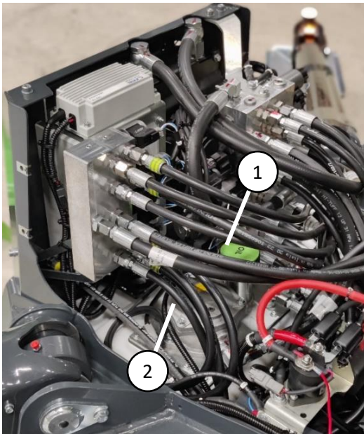
Kuva 22. Paluusuodattimen sijainti
