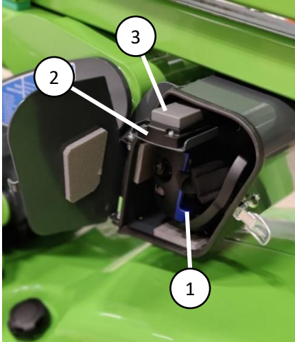
Kuva 5. Kauko-ohjaimen säilytyskotelo
