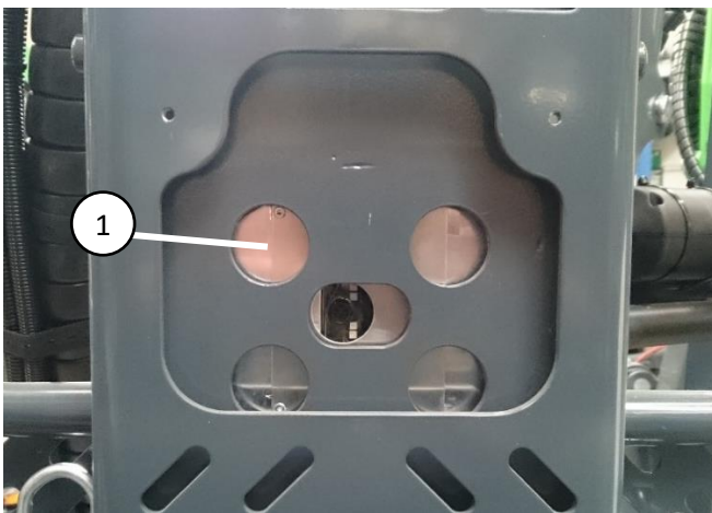
Kuva 36. Kuorma-anturi
