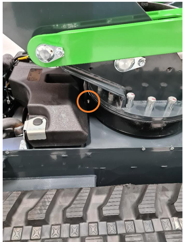
Kuva 17. Kääntökehän rasvauspaineen vapautusruuvi
