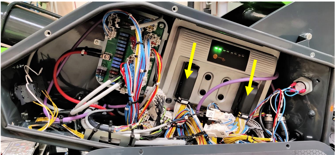
Kuva 45. Logiikkaohjaimien liittimet (2 kpl), osoitettu nuolella
