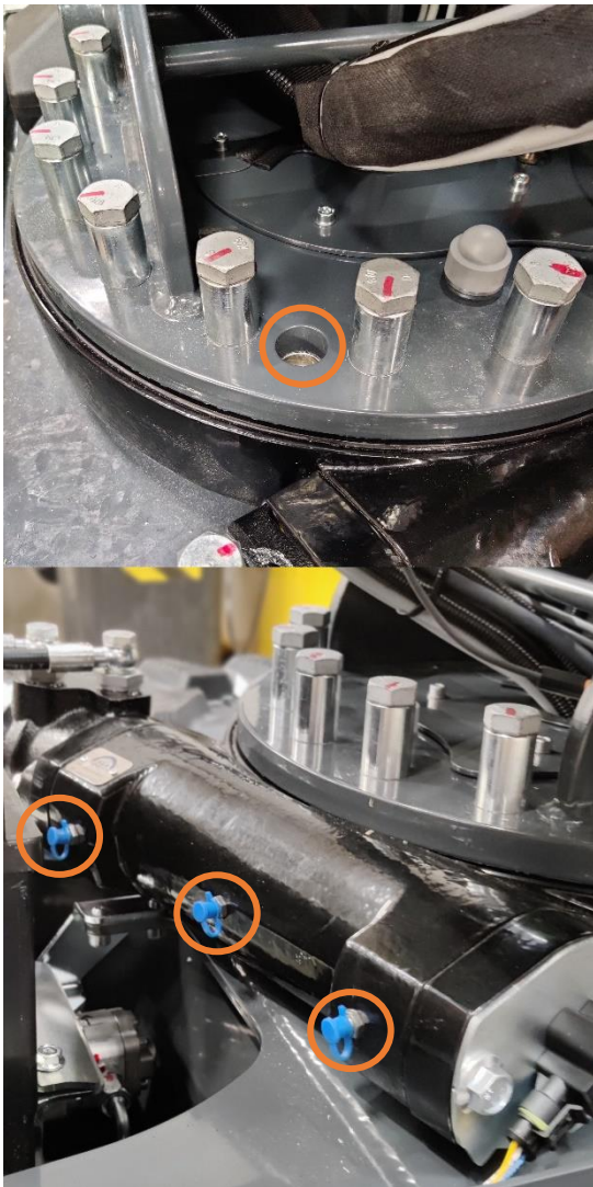
Kuva 16. Kääntökehän voitelupisteet
