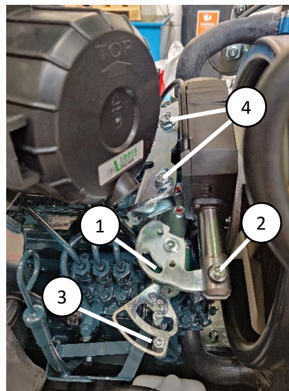
Kuva 27. Kaasunsäätömoottorin maksimiasento
