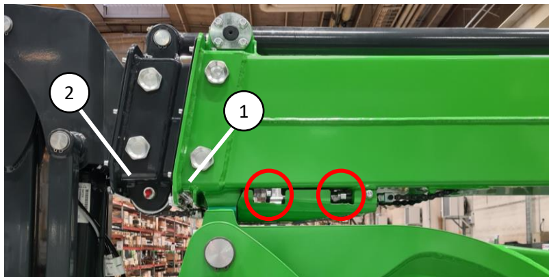
Kuva 13. Teleskoopin ketjun kirityksen osoittimet ja liukupalat
