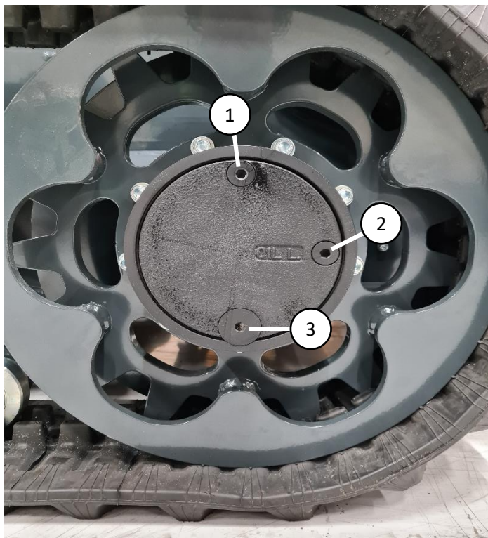
Kuva 25. Ajomoottorin vaihteiston öljynvaihto
