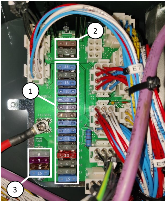
Kuva 43. Laitteen sulakkeet
