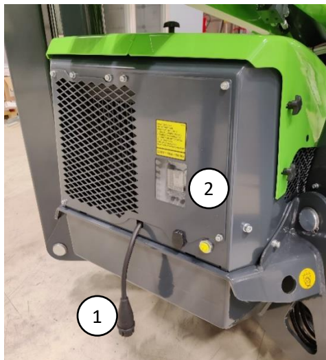
Kuva 7. 230 V kytkennät
