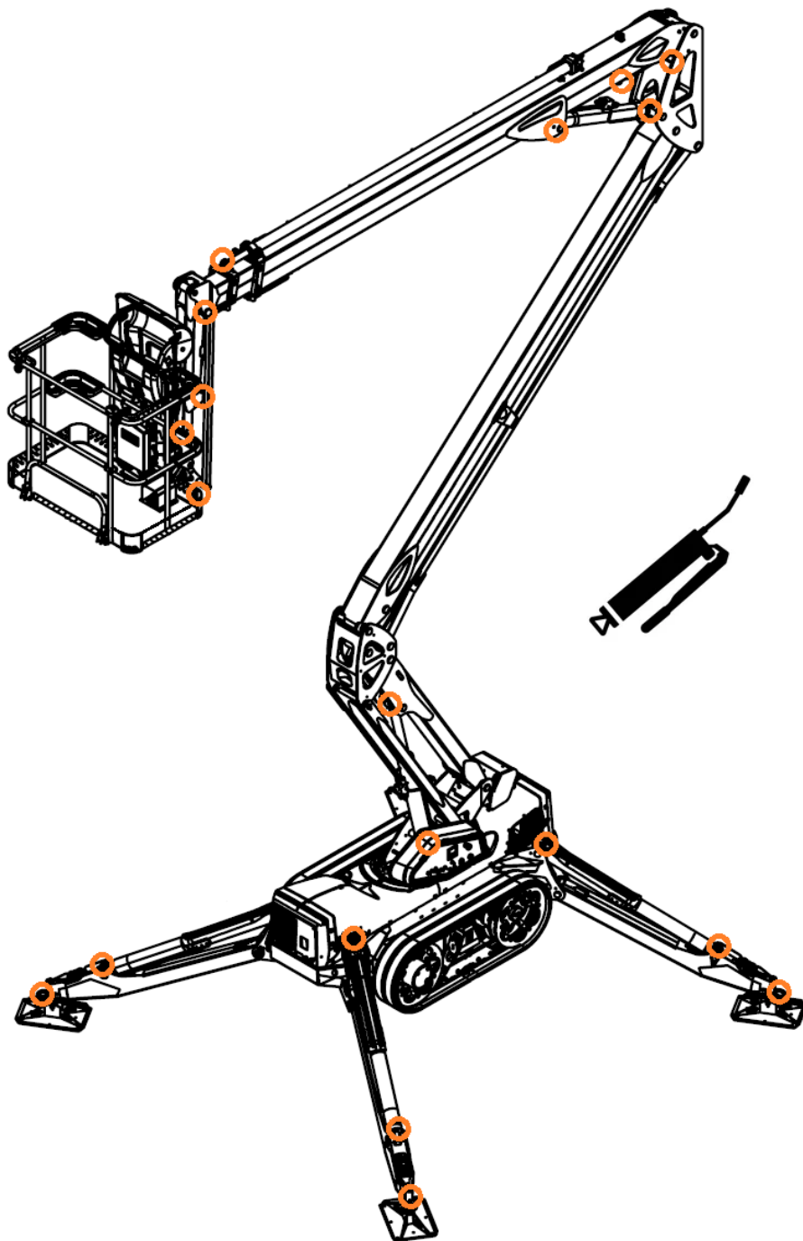
Kuva 15. Voitelukaavio
