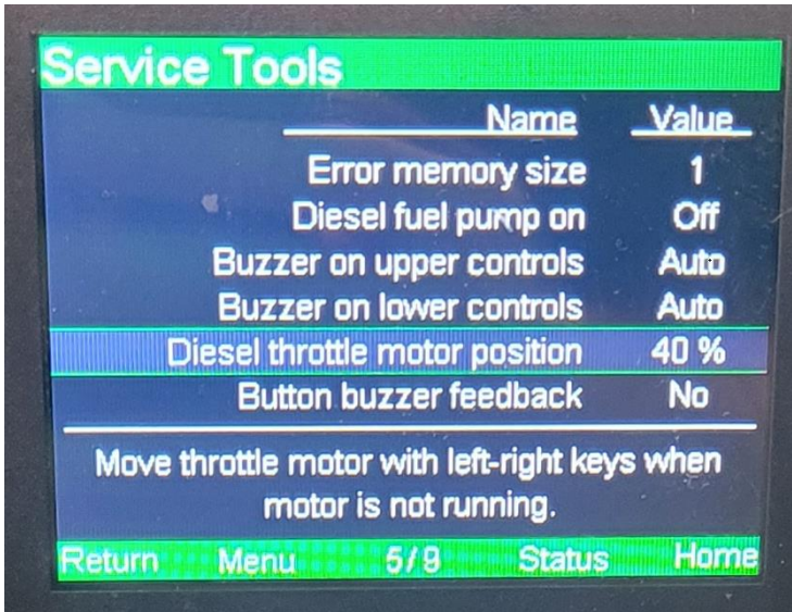
Kuva 29. Kaasunsäätömoottorin asento jarrua säädettyä
