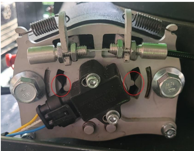
Kuva 30. Jarruvaijerin säätö
