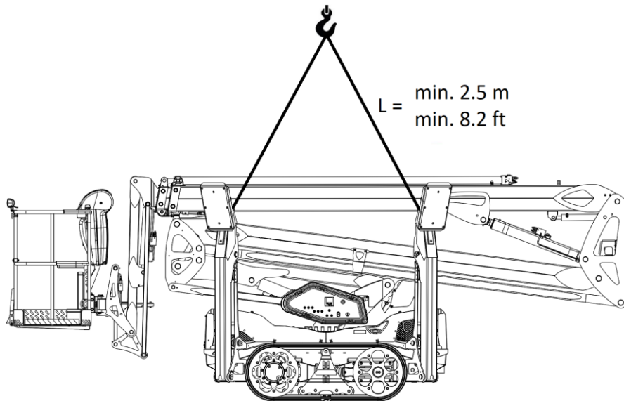
Kuva 10. Tukijalkojen nostopisteet
