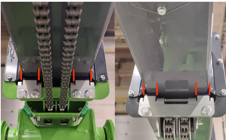
Kuva 20. Välipuomin ja jatkeen rasvattavien liukupintojen reunaviivat rajattu punaisella.
