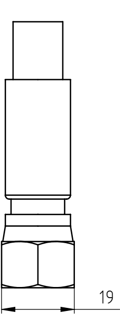
JIC 9/16
