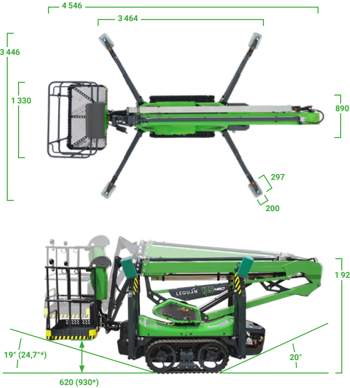
Mitat millimetreinä. *Korotetun ajoasennon (EDP) enimmäisarvot.
