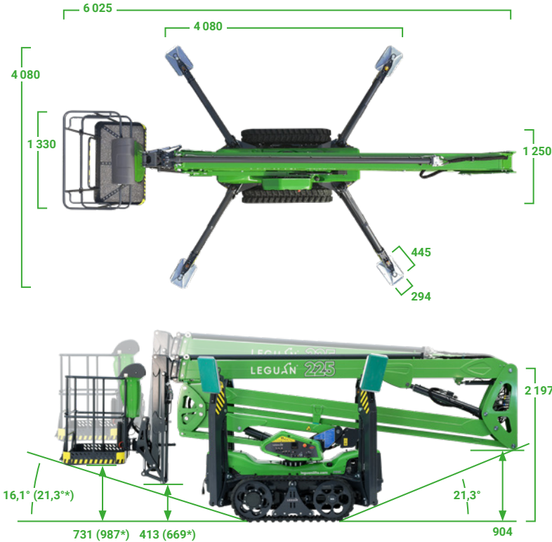
Mitat millimetreinä. *Korotetun ajoasennon (EDP) enimmäisarvot.
